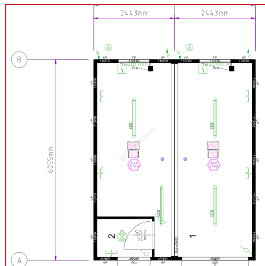
Beispiel: Container - Skizze 6x5 m, andere Größen möglich
